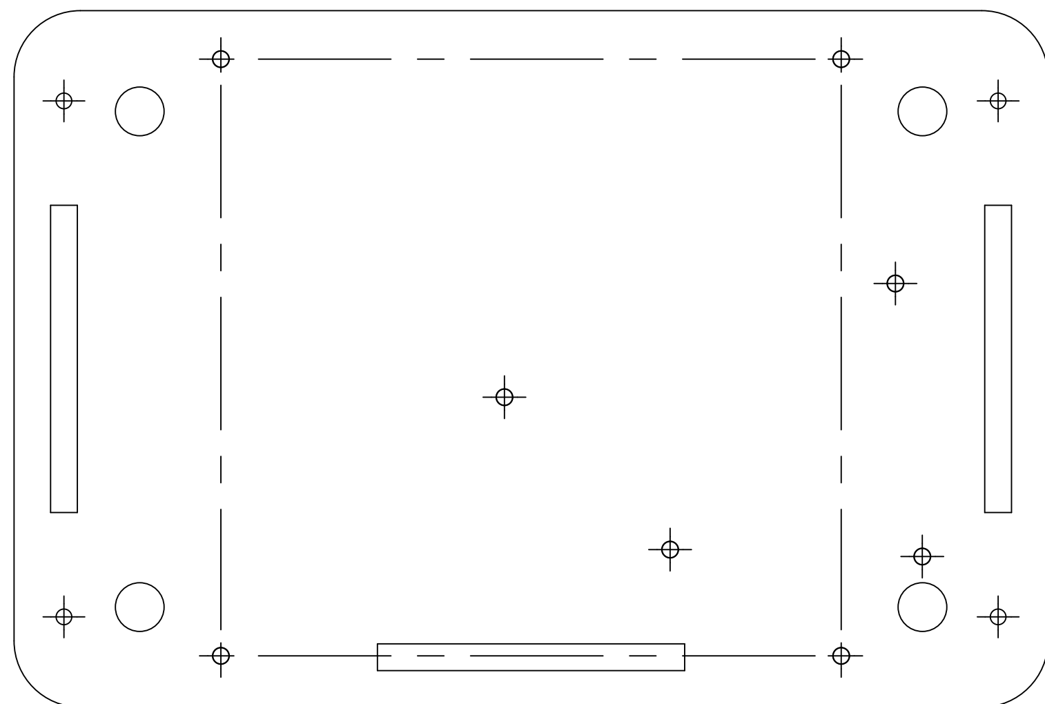
Body Bottom
